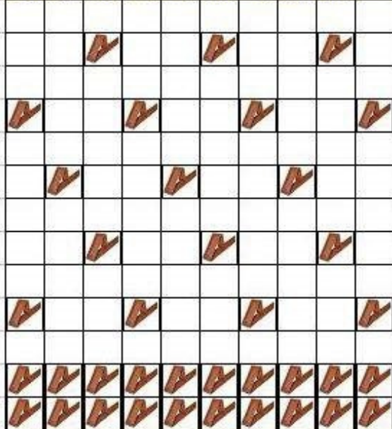
Verlegebeispiel bei ca. 3 Stück je m2
